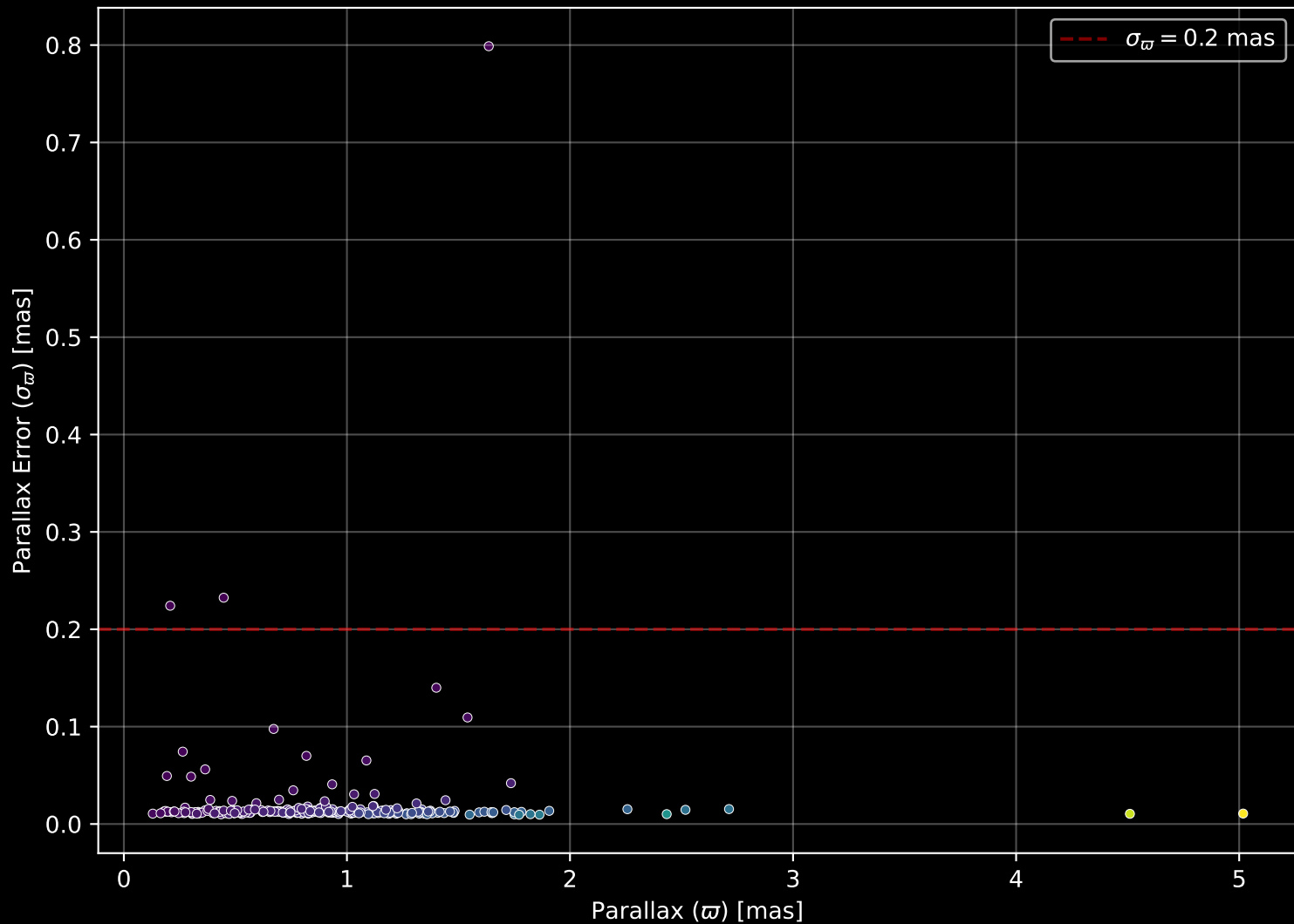
GALAH DR4 Field: [8435] Parallax Quality (n= 235)
