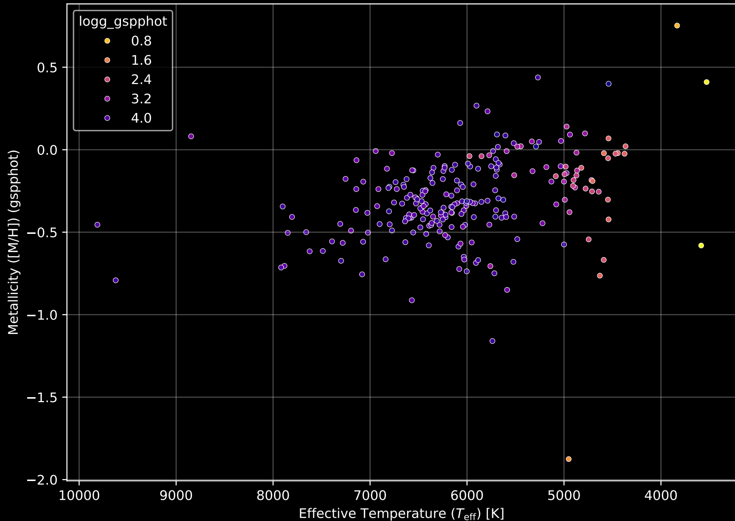
GALAH DR4 Field: [8435] Stellar Population Parameters (n= 235)
