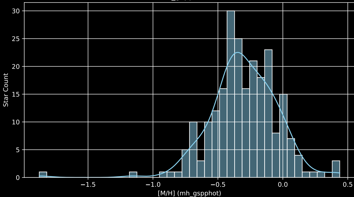
GALAH DR4 Field: [8435] [M/H] (mh_gspphot) (n= 234)
