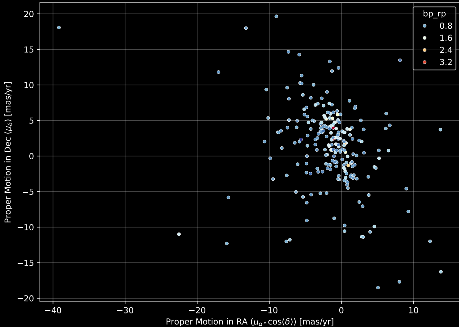
GALAH DR4 Field: [8435] Proper Motion Diagram (n= 235)
