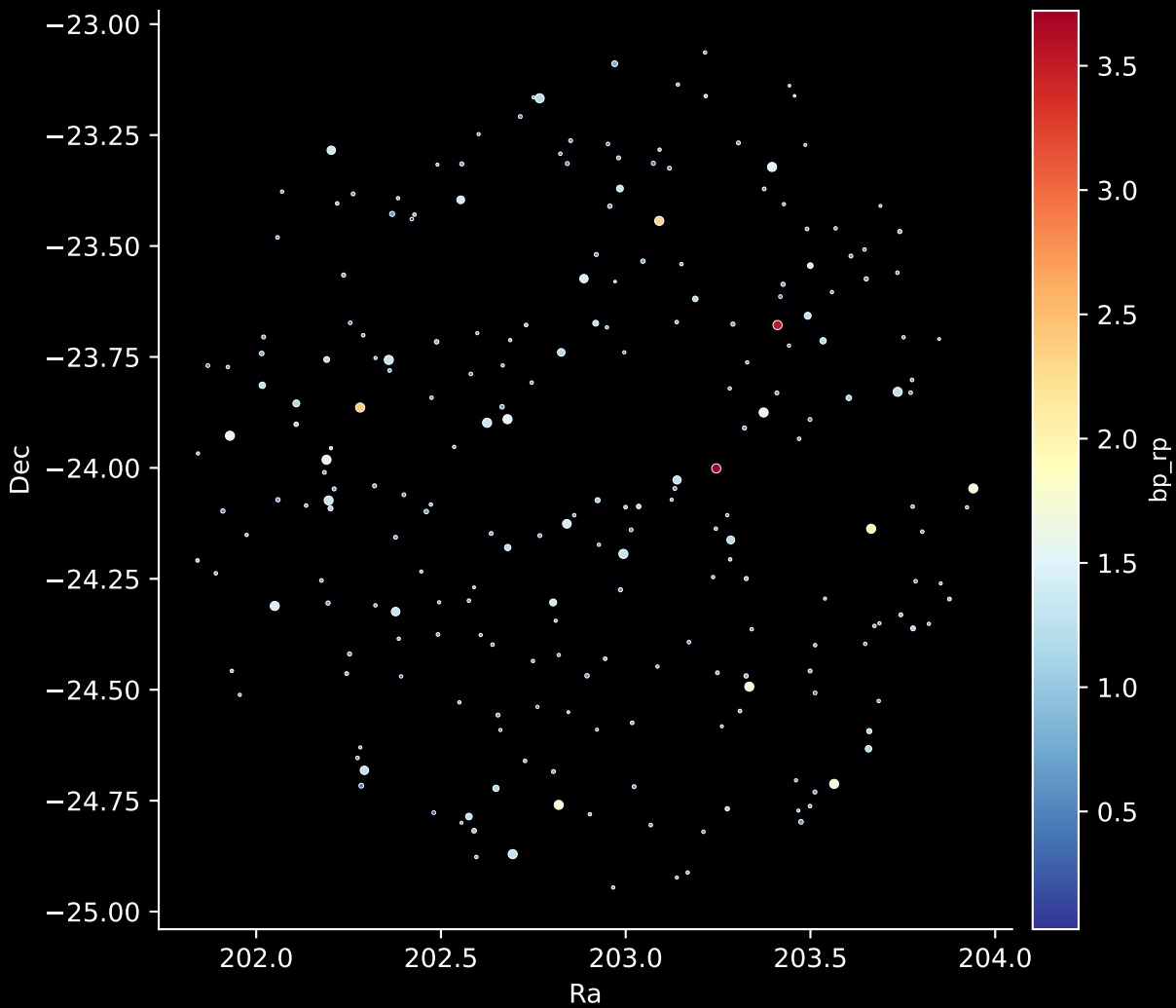
GALAH DR4 Field: [8435] Stars: 235
